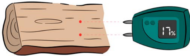
Zwei Elektroden werden in das Holz eingeschlagen. Der Widerstand beim Stromfluss ist für den Restwassergehalt bezeichnend.
